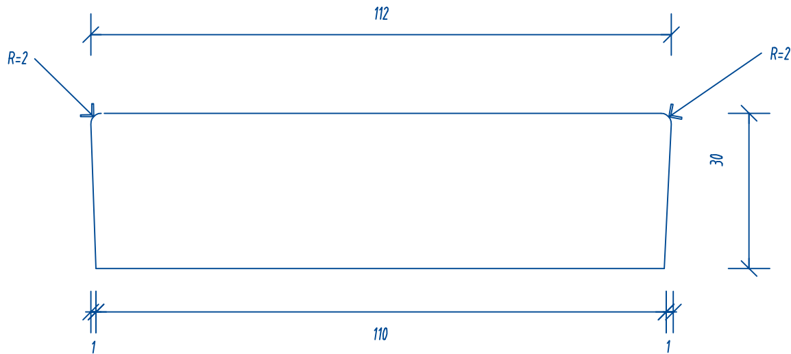
IJSP-112x30 Primed Radiata FJ Door Jamb/Head
